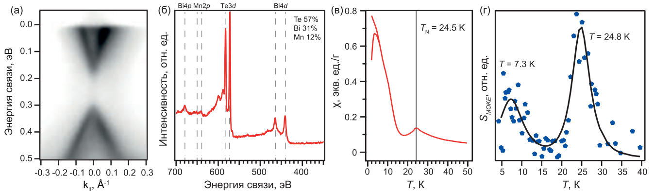
Рис. 1. \text{MnBi}_2\text{Te}_4 : а – ФЭСУР дисперсионная зависимость, измеренная в точке \Gamma , б – РФЭС-спектр остовных уровней элементов, присутствующих в образце, положения уровней отмечены вертикальными линиями, в – зависимость магнитной восприимчивости от температуры, температура АФМ-упорядочения отмечена вертикальной линией, г – зависимость S_{\text{МОКЕ}}(T) представлена точками, аппроксимация сигнала пиками Гаусса отмечена кривой.
