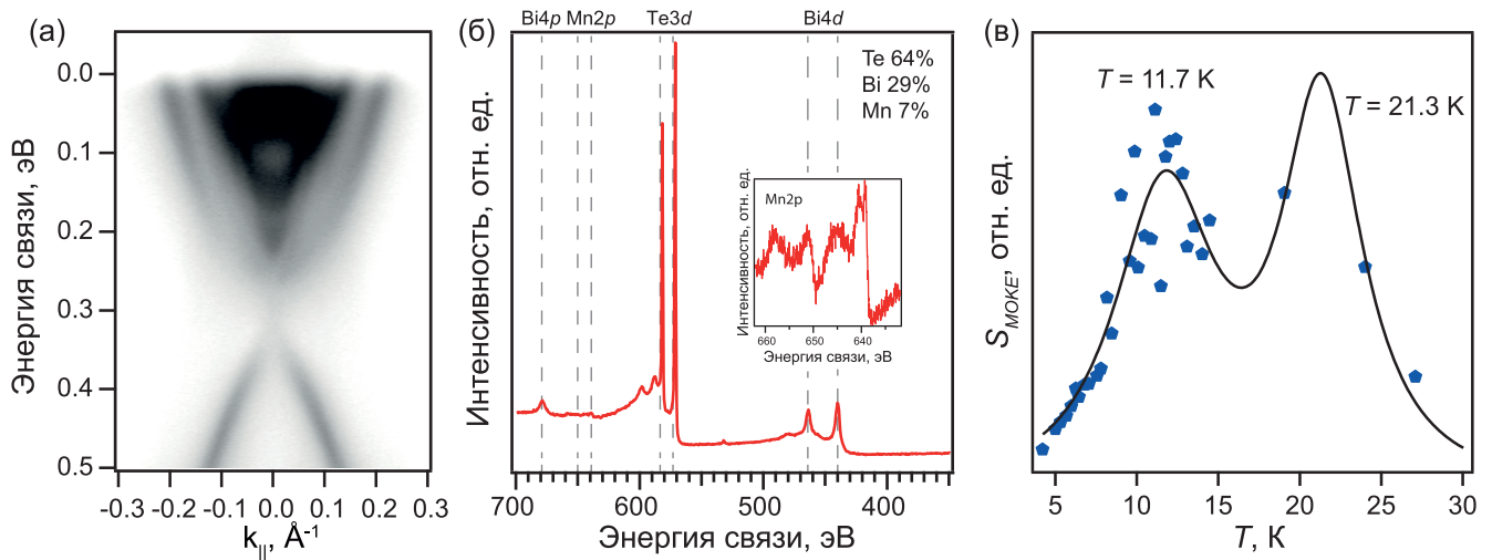
Рис. 2. \text{MnBi}_2\text{Te}_4 : а – ФЭСУР дисперсионная зависимость, измеренная в точке \Gamma , б – РФЭС-спектр остовных уровней элементов, присутствующих в образце, положения уровней отмечены вертикальными линиями. На вставке – область 2p -уровня Mn; в – зависимость S_{\text{MOKE}}(T) представлена точками, аппроксимация сигнала пиками Гаусса отмечена кривой.
