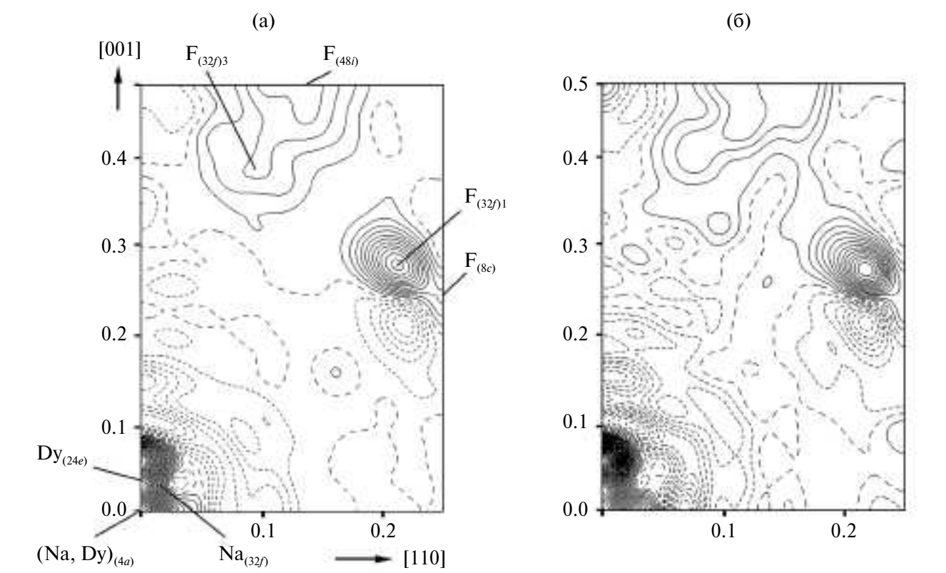
Рис. 2. Разностные карты Фурье электронной плотности α-Na 0.35 Dy 0.65 F 2.30 в плоскости (110) при 293 (а) и 85 К (б). Шаг изолиний 0.2 Å −3 .
