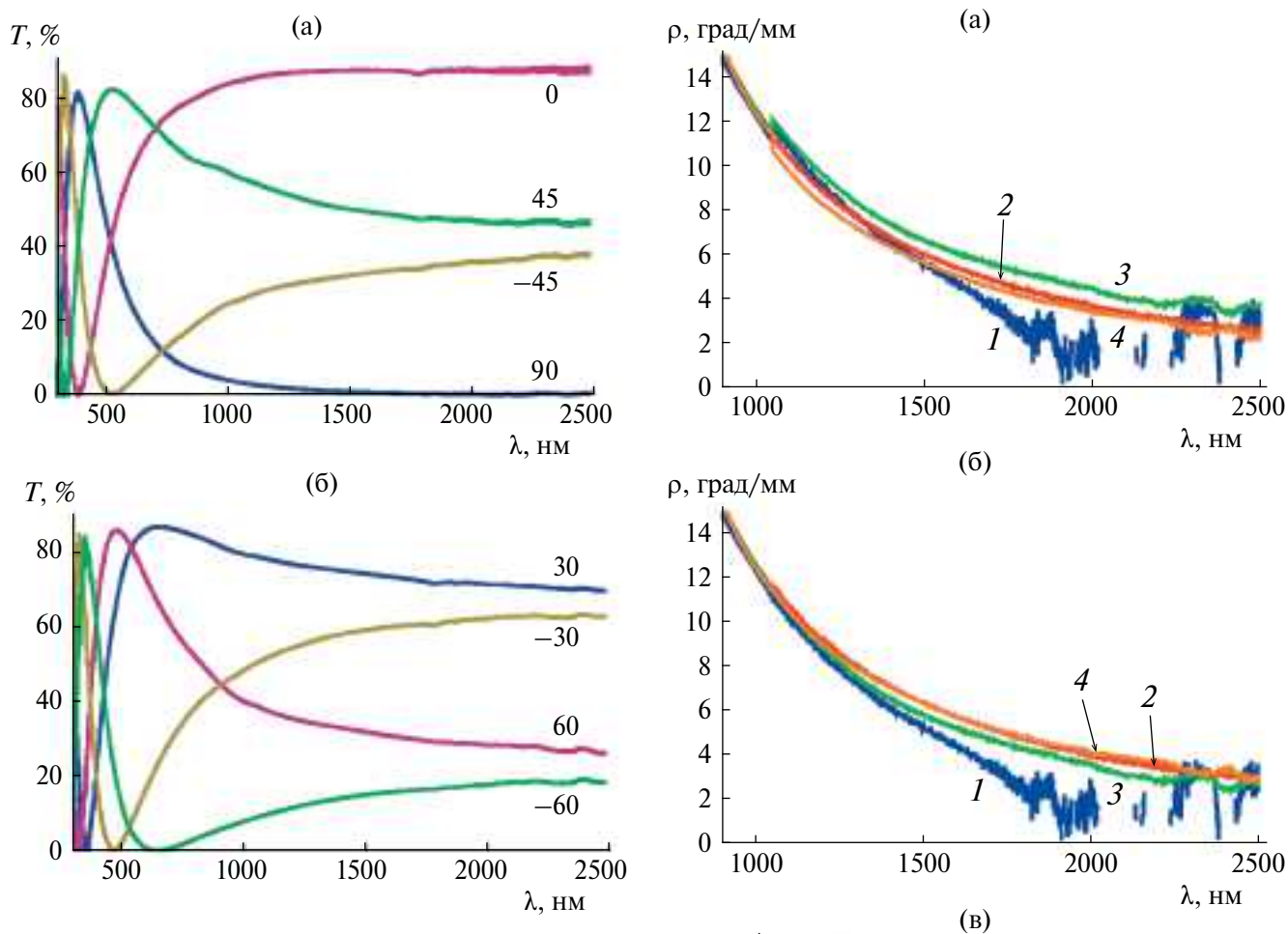
Рис. 3. Нормированные спектры коэффициентов пропускания для образца 1, нормировка проводилась делением части спектра при \lambda > 1050 нм на величину h = T(1050 \text{ нм})/T(1049 \text{ нм}) .
