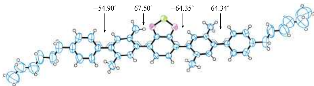
Рис. 5. Конформация молекулы Нех-Ph-Ху-ВТД в ORTEP-представлении с указанием торсионных углов между сопряженными группами (тепловые эллипсоиды с вероятностью на уровне 50%).
