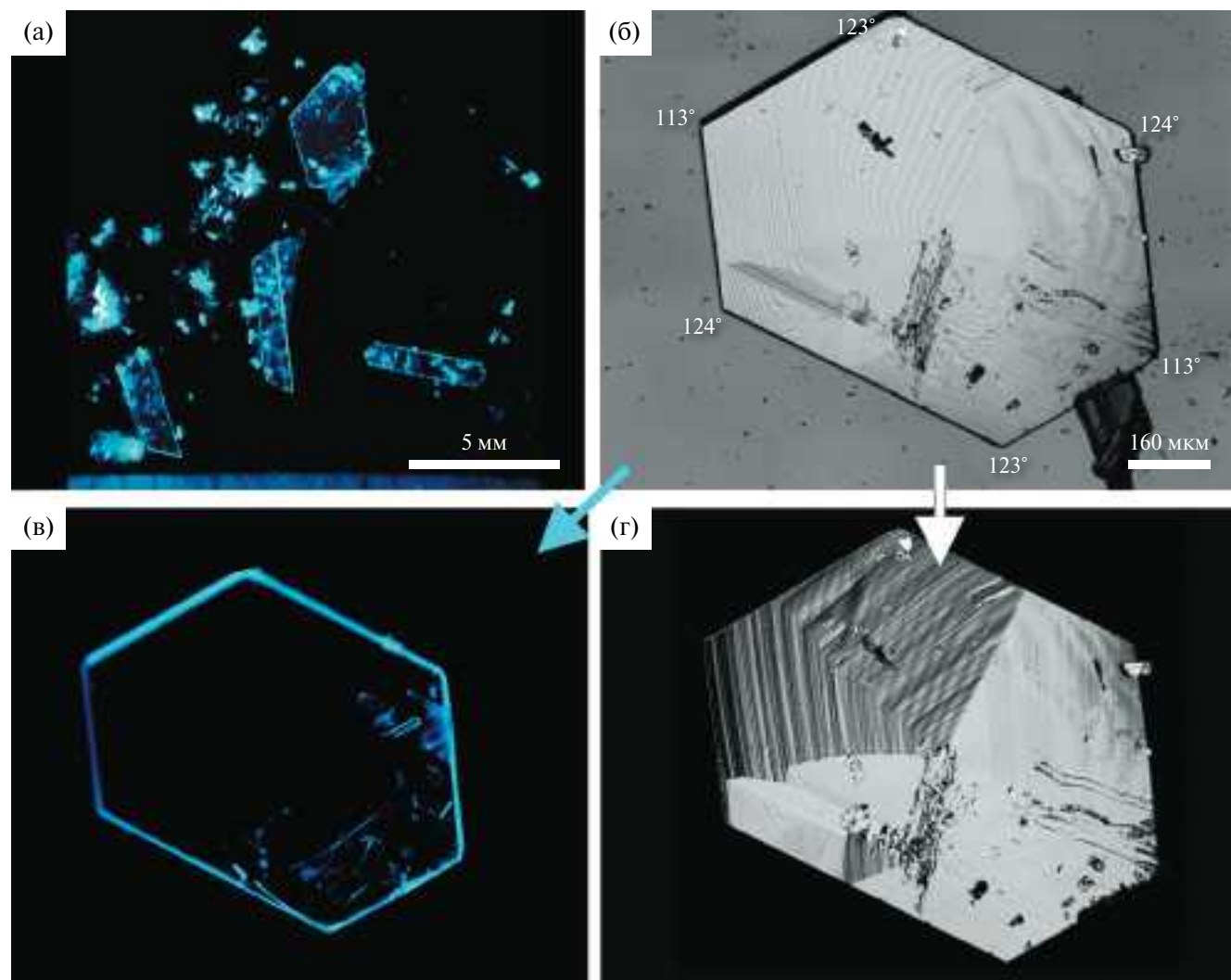
Рис. 4. Кристаллы Нех-Ph-Ху-ВТД: под УФ-освещением (а), конфокальное изображение ограненного кристалла (б) и его изображения в люминесцентном режиме (в) и в режиме дифференциально-интерференционного контраста (г).
