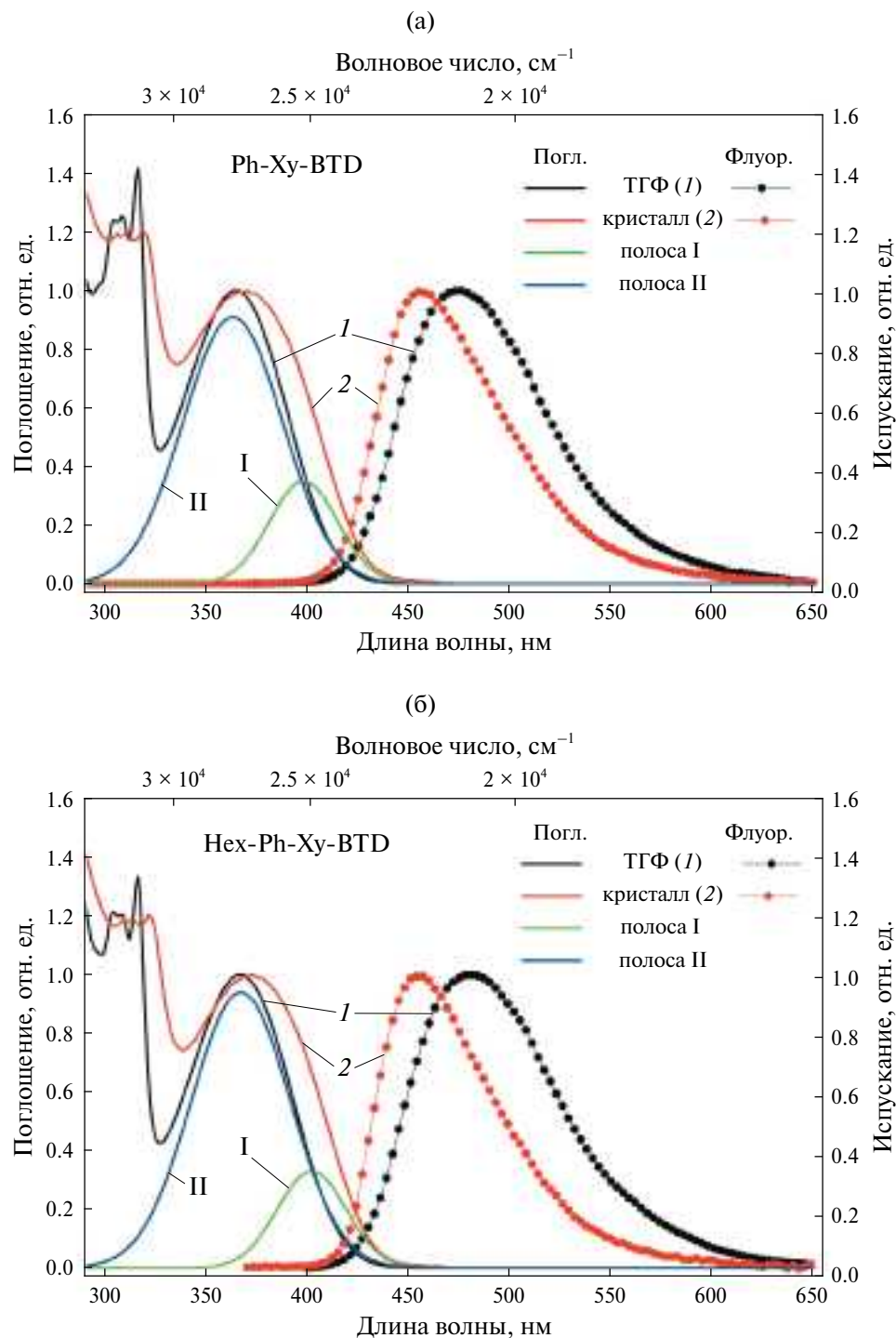
Рис. 9. Нормированные спектры поглощения и флуоресценции Ph-Ху-ВТД (а) и Нех-Ph-Ху-ВТД (б) в растворе ТГФ и в тонкой поликристаллической пленке (без реабсорбции). Выделение полосы поглощения центров флуоресценции (полоса I) в тонкой поликристаллической пленке. Возбуждение осуществлялось в длинноволновом максимуме поглощения.
