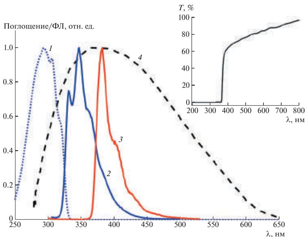
Рис. 7. Нормированные спектры оптического поглощения (1) и фотолюминесценции (2) раствора транс -стильбена в n -гексане; спектр ФЛ монокристалла транс -стильбена толщиной d_1 = 1 мм (3); аппаратная функция фотокатода детектора R10131 в единицах квантовой эффективности (4). На вставке в правом верхнем углу изображения – спектр пропускания образца на основе монокристалла транс -стильбена ( d_2 = 5 мм).
